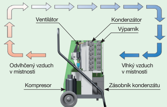
Schématické znázornění principu činnosti
